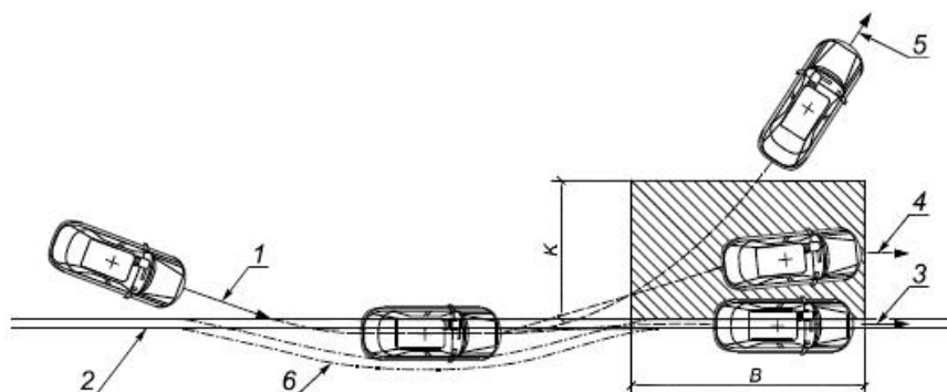
Рисунок 4 - Границы коридора выбега ТС после наезда на ограждение
